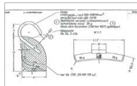
Technische Zeichnung für Schlaggewichte
