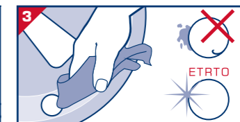
Das Ventilloch muss frei von Schmutz und Graten sein und muss der ETRTO entsprechen
